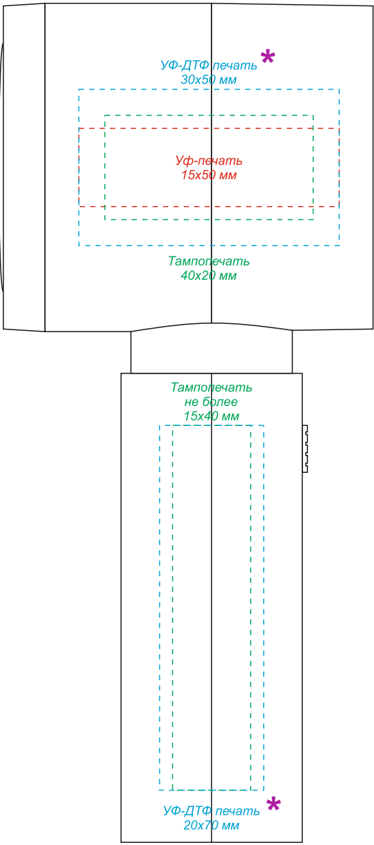
Вид слева
