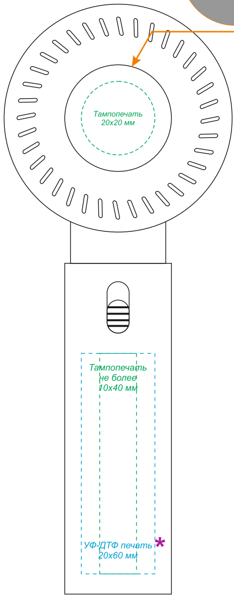
Вид сзади
