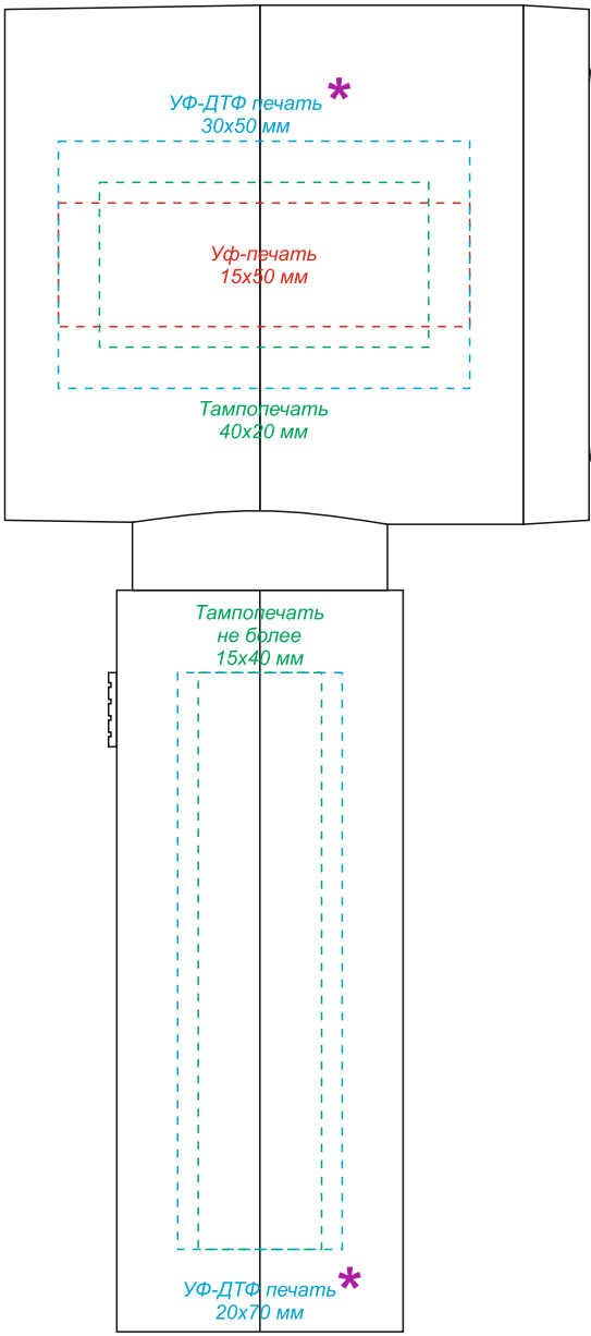
Вид справа
